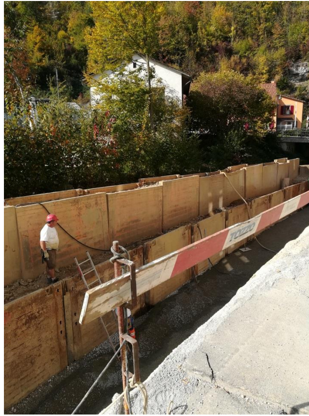
Fundamente für die neue Bachmauer
