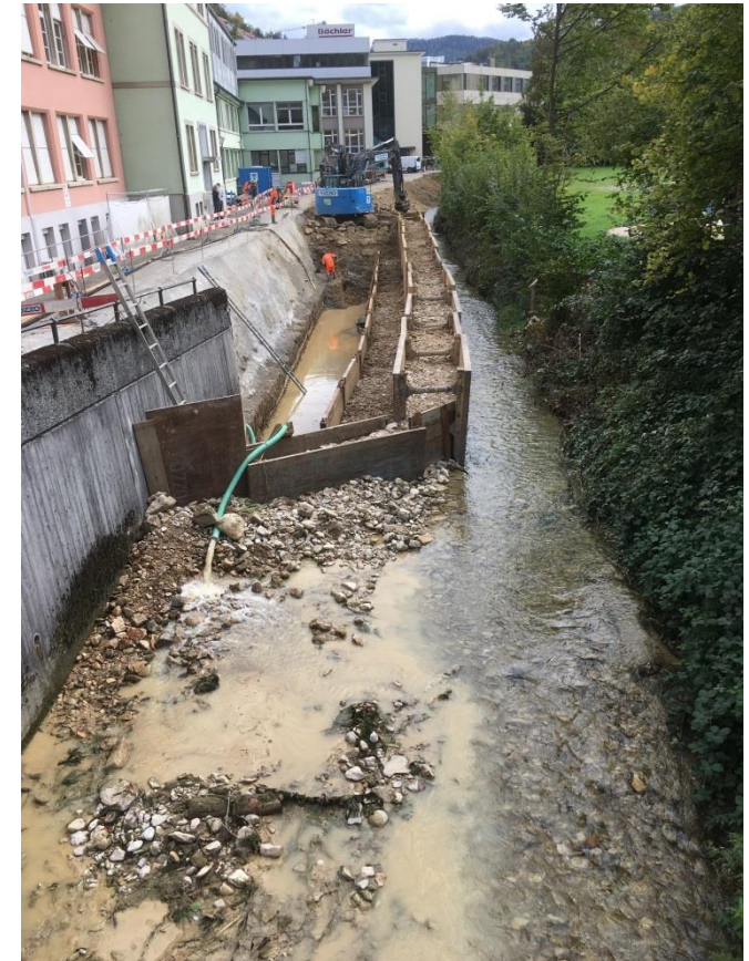
Ribigasse aus Richtung Hauptstrasse Baugrube auf Höhe Oris
