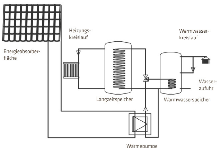
Abbildung 1: Schema des Metallziegel-Wärmepumpensystems
