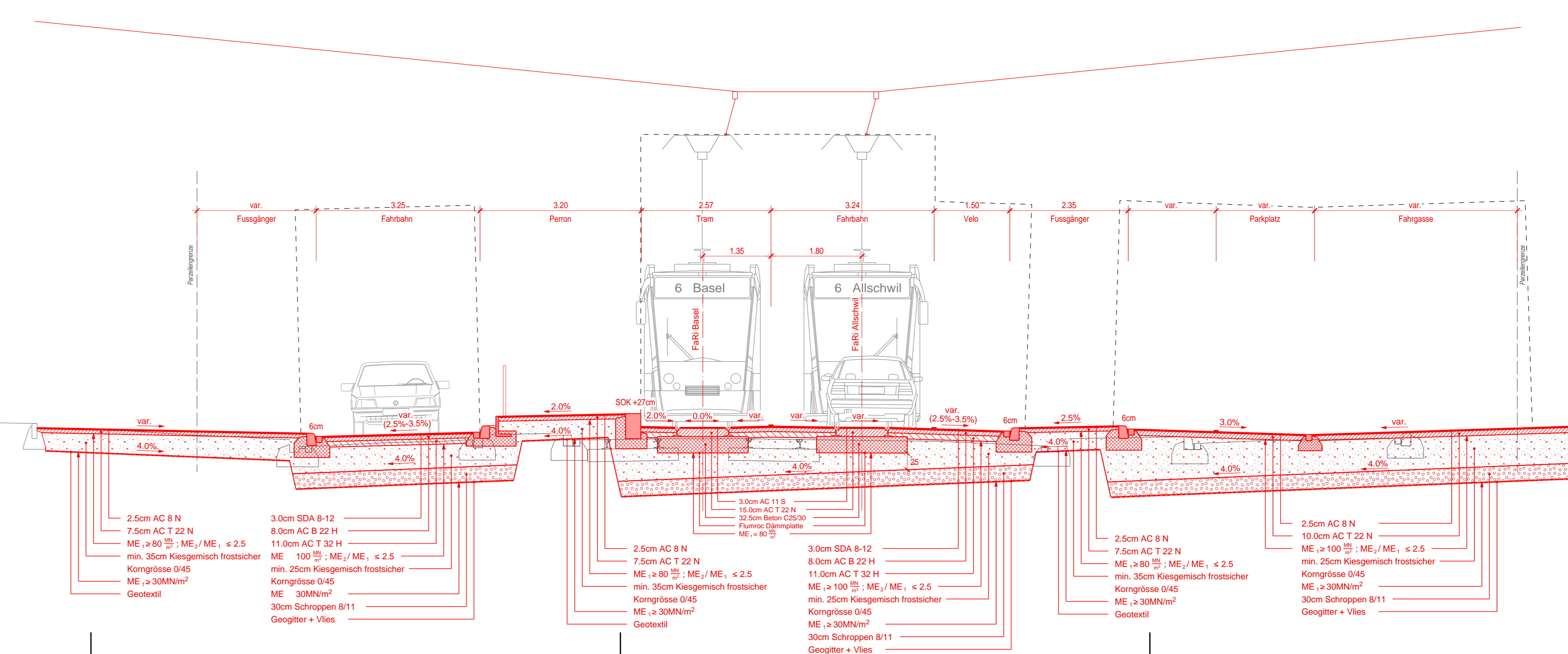
Normalprofil 4
