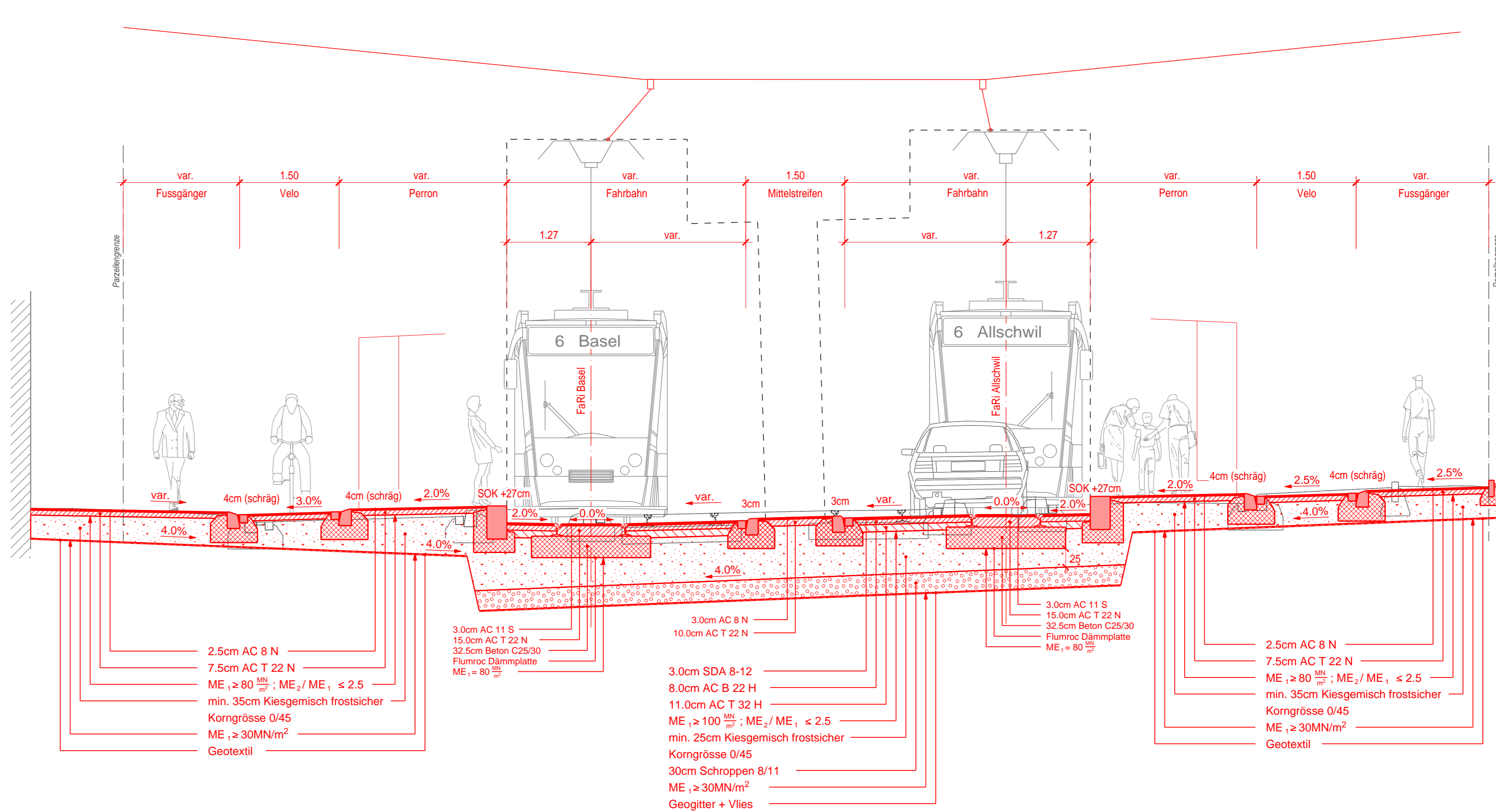
Normalprofil 2
