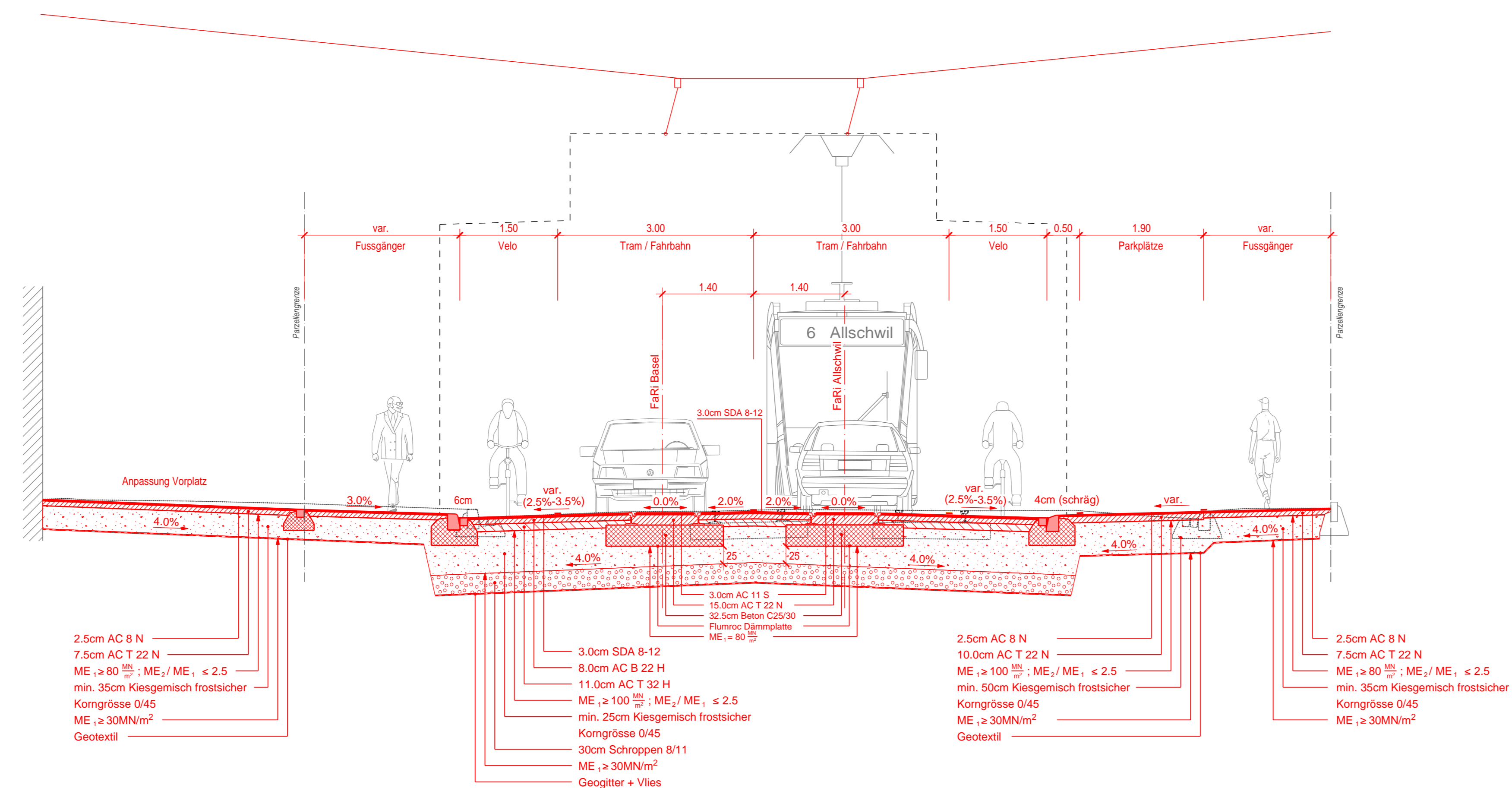
Normalprofil 1
