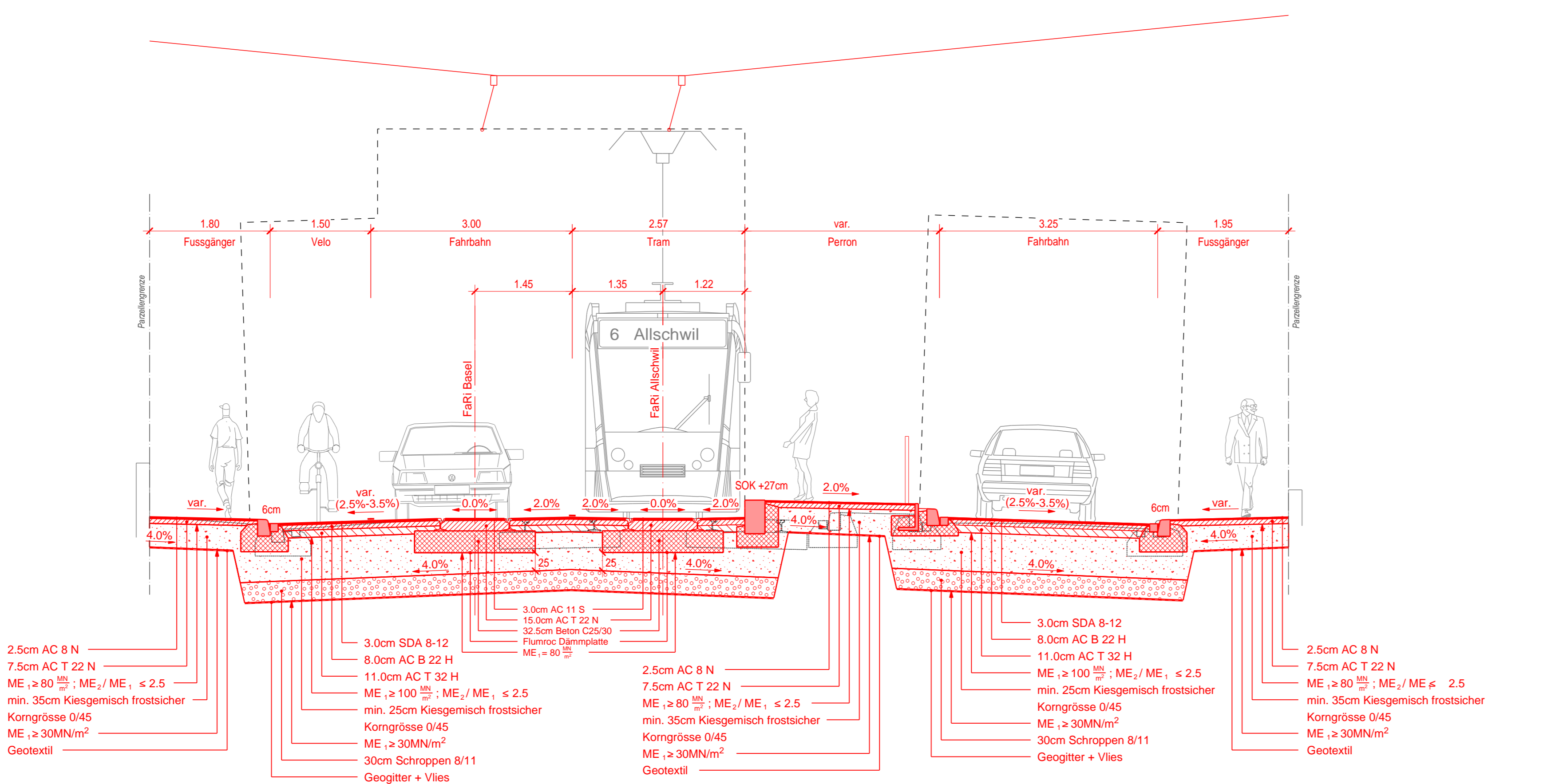
Normalprofil 3
