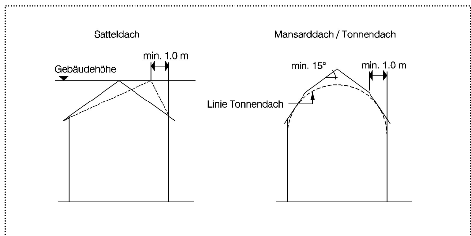
Prinzipskizze Firstanordnung
