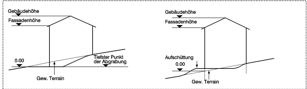
Messpunkte
