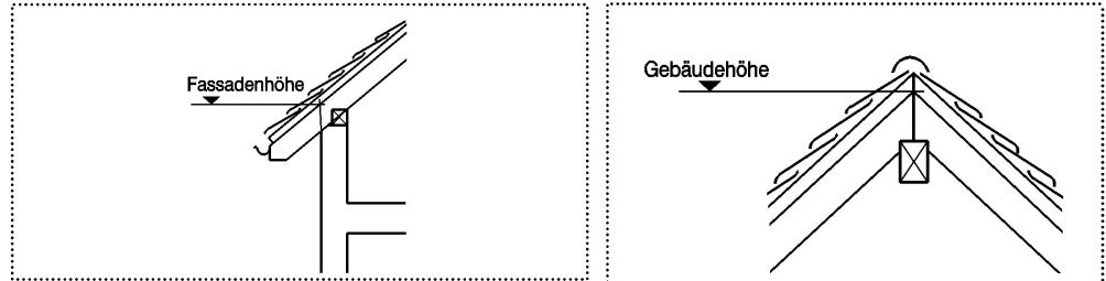
Messpunkte
