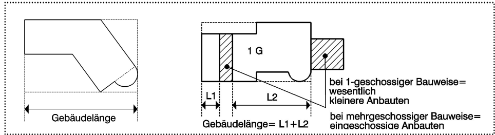
Prinzipskizze Gebäudelänge
