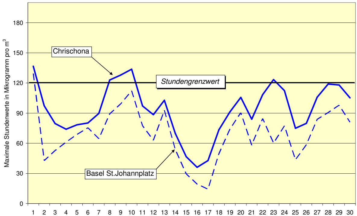
Ozon (O 3 ): Verlauf der täglichen maximalen Stundenwerte im September 2009
