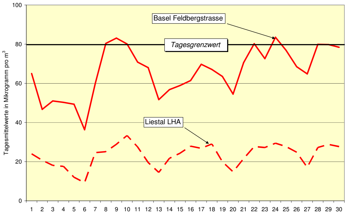
Stickstoffdioxid (NO 2 ): Verlauf der Tageswerte im September 2009
