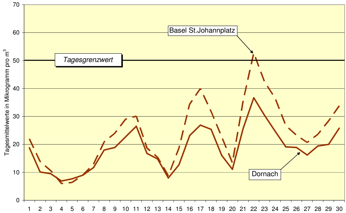
Feinstaub (PM10): Verlauf der Tageswerte im September 2009
