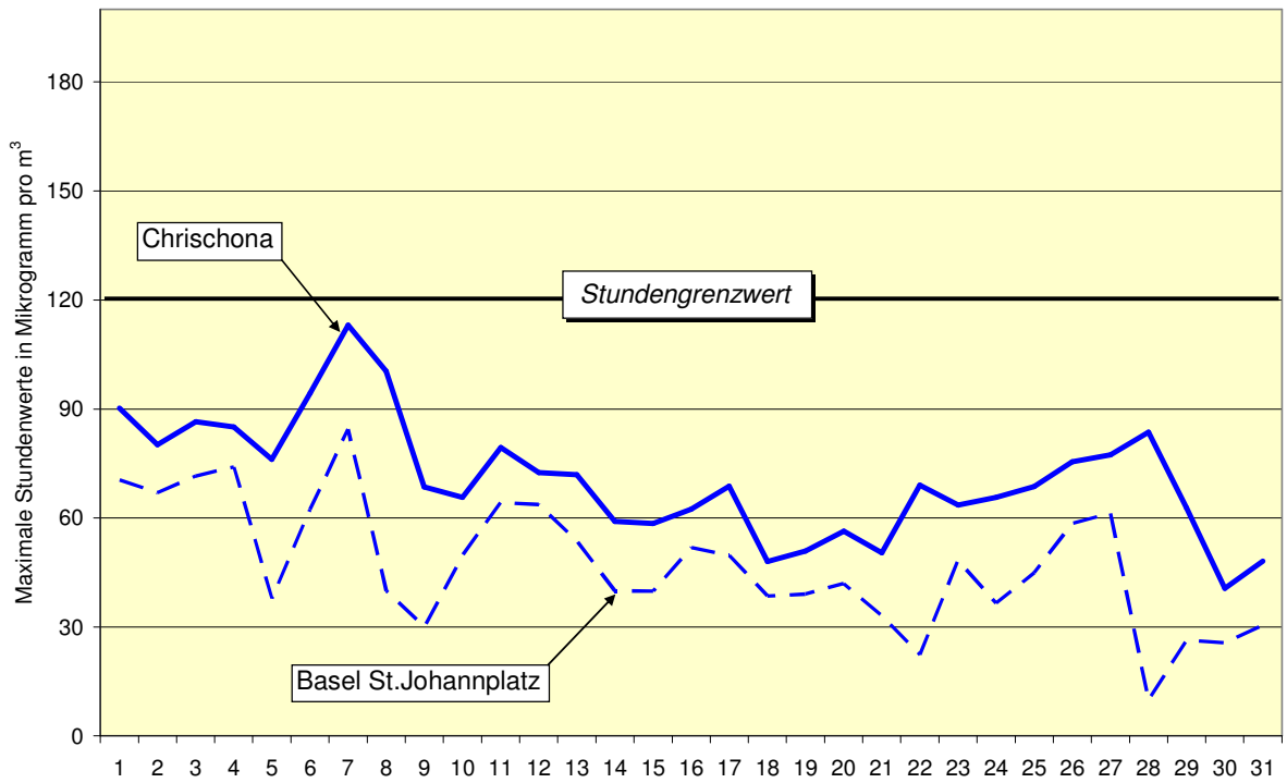
Ozon (O 3 ): Verlauf der täglichen maximalen Stundenwerte im Oktober 2009
