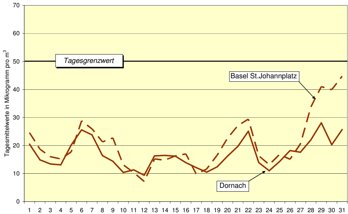
Feinstaub (PM10): Verlauf der Tageswerte im Oktober 2009
