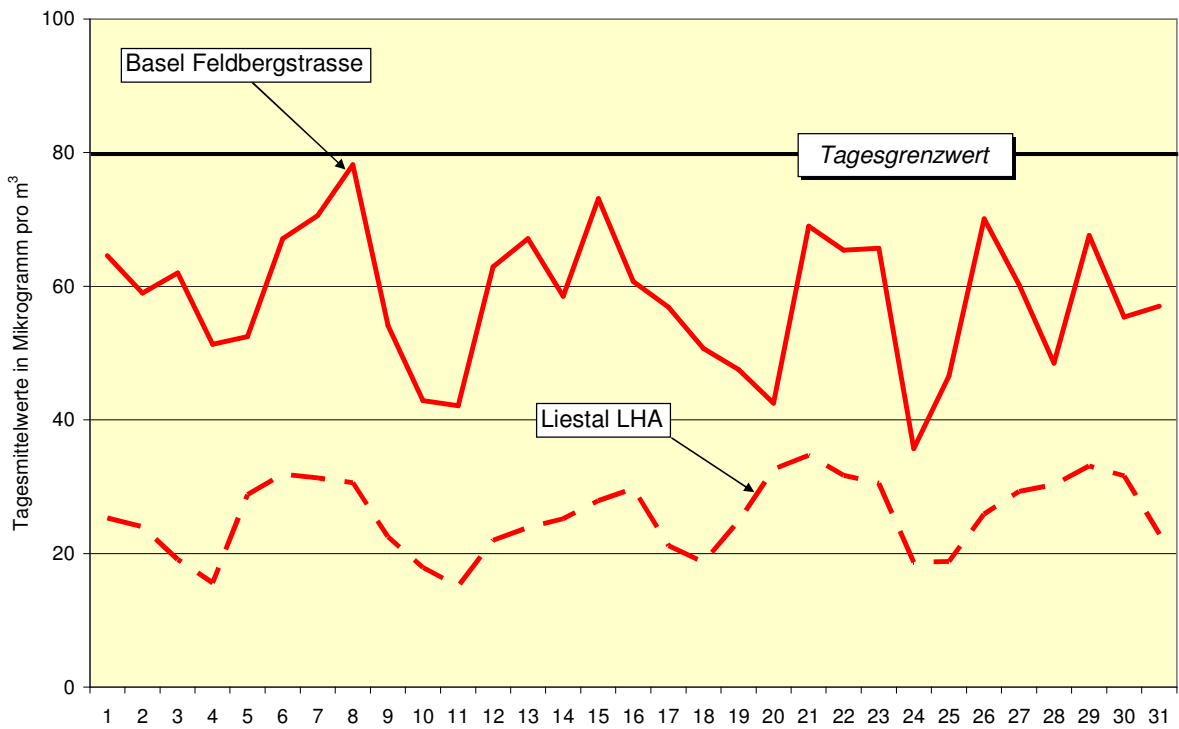
Stickstoffdioxid (NO 2 ): Verlauf der Tageswerte im Oktober 2009
