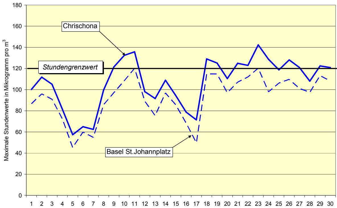
Ozon (O 3 ): Verlauf der täglichen maximalen Stundenwerte im Juni 2008
