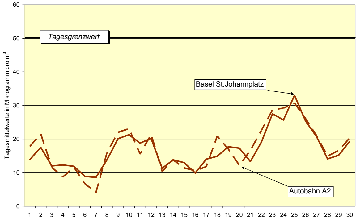
Feinstaub (PM10): Verlauf der Tageswerte im Juni 2008
