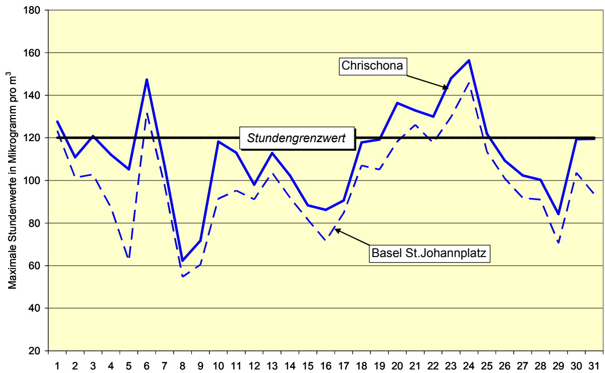
Ozon (O 3 ): Verlauf der täglichen maximalen Stundenwerte im Mai 2007
