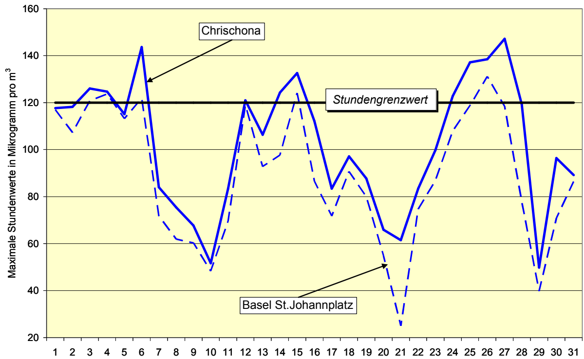
Ozon (O 3 ): Verlauf der täglichen maximalen Stundenwerte im August 2007
