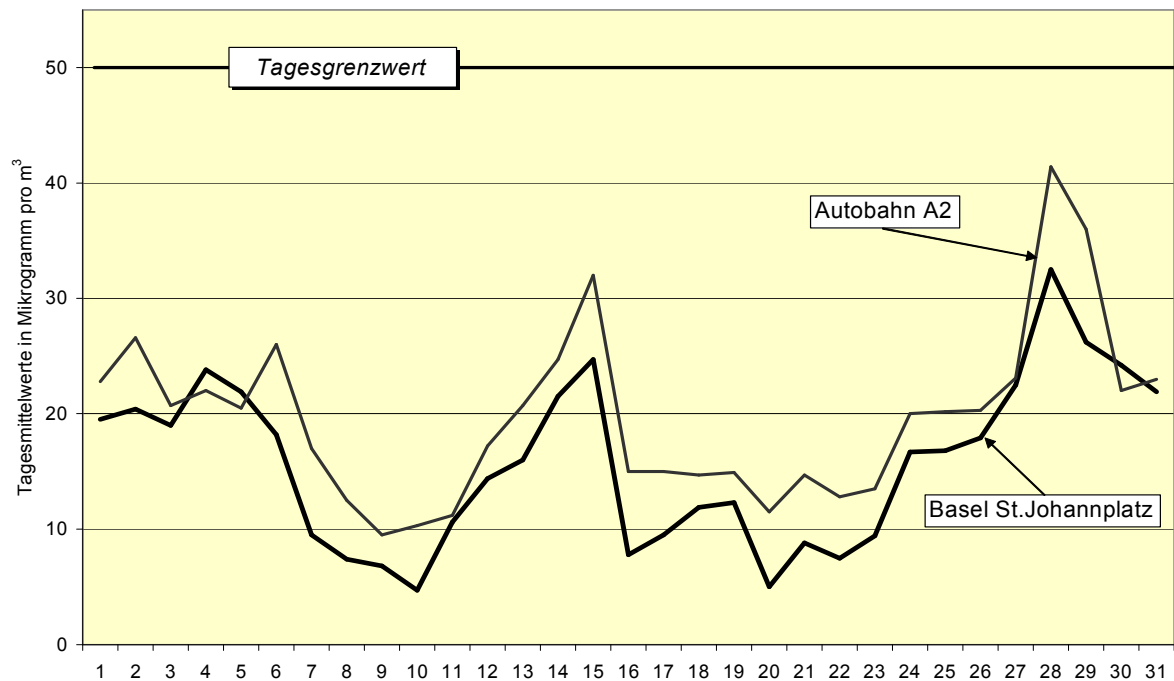
Feinstaub (PM10): Verlauf der Tageswerte im JAugust 2007
