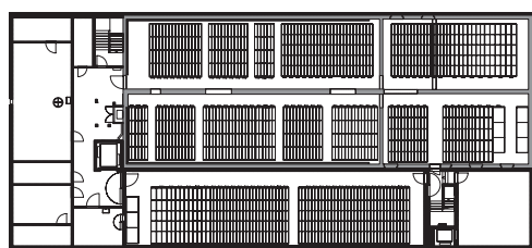
Untergeschoss
