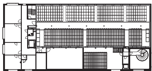
1. Obergeschoss
